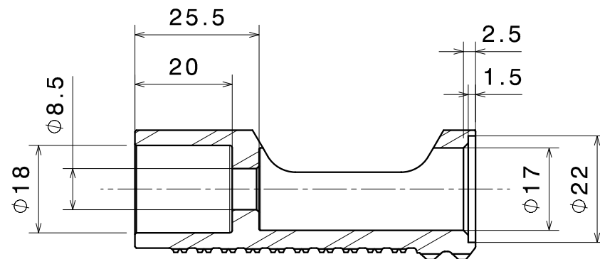
Vista in sezione A-A
