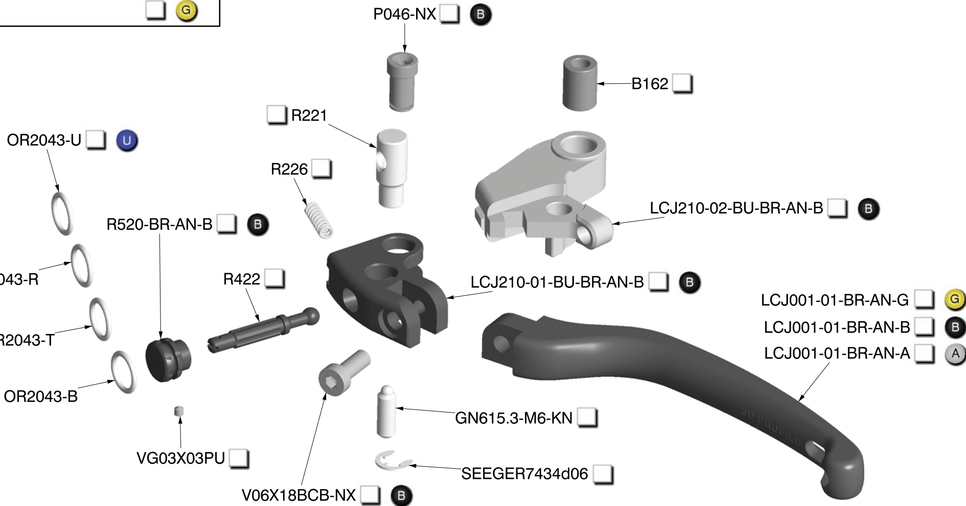
LCJ210 (Leva frizione completa) (Complete clutch lever)
